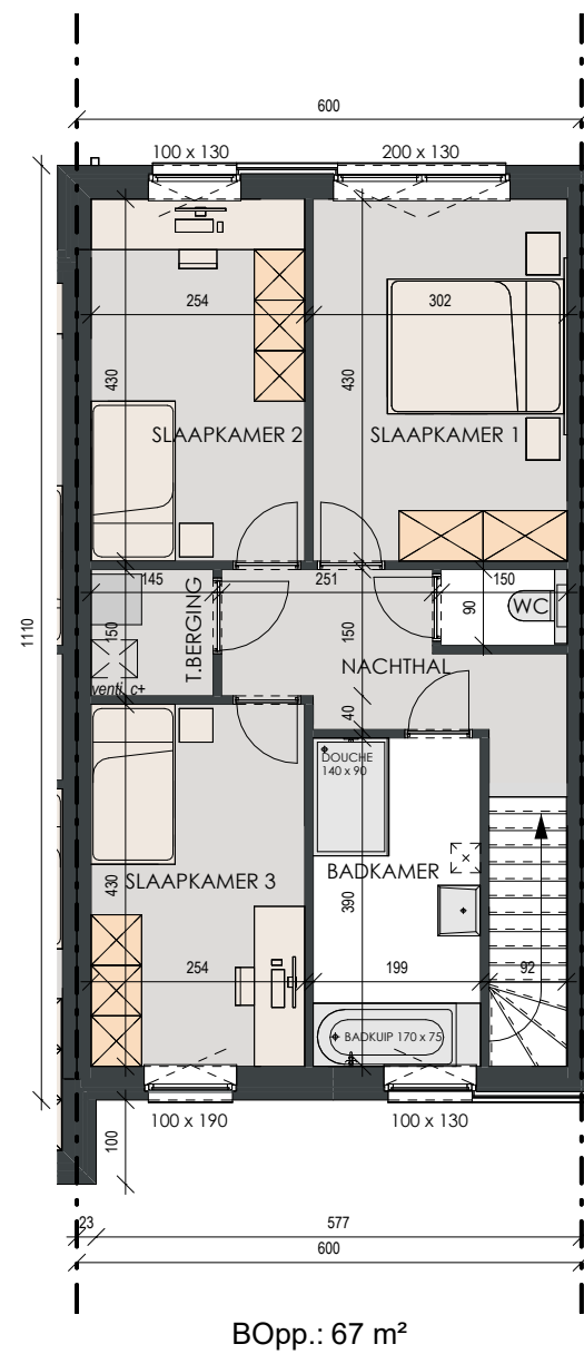
1e Verdieping 1:100
