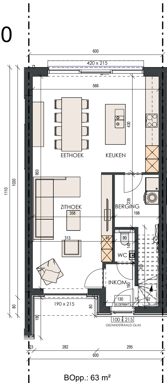
Gelijkvloers 1:100
